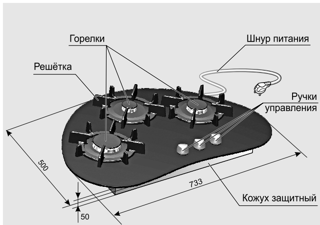
Рис. 1 МОДЕЛЬ СН2120
