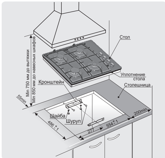
Рис. 5 МОДЕЛЬ СВН2230; -01
