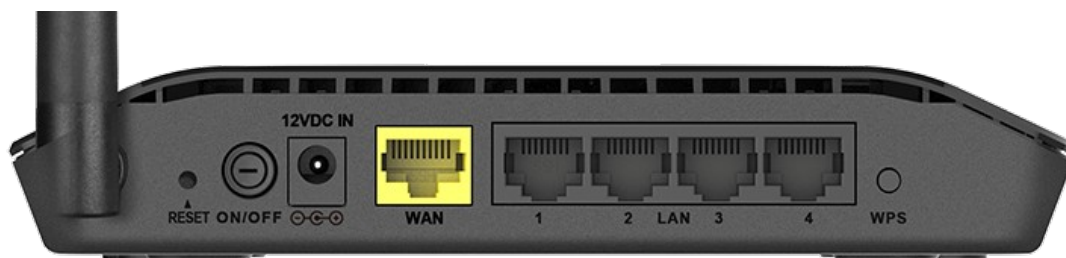
Рисунок 2. Вид задней панели DIR-300S.
